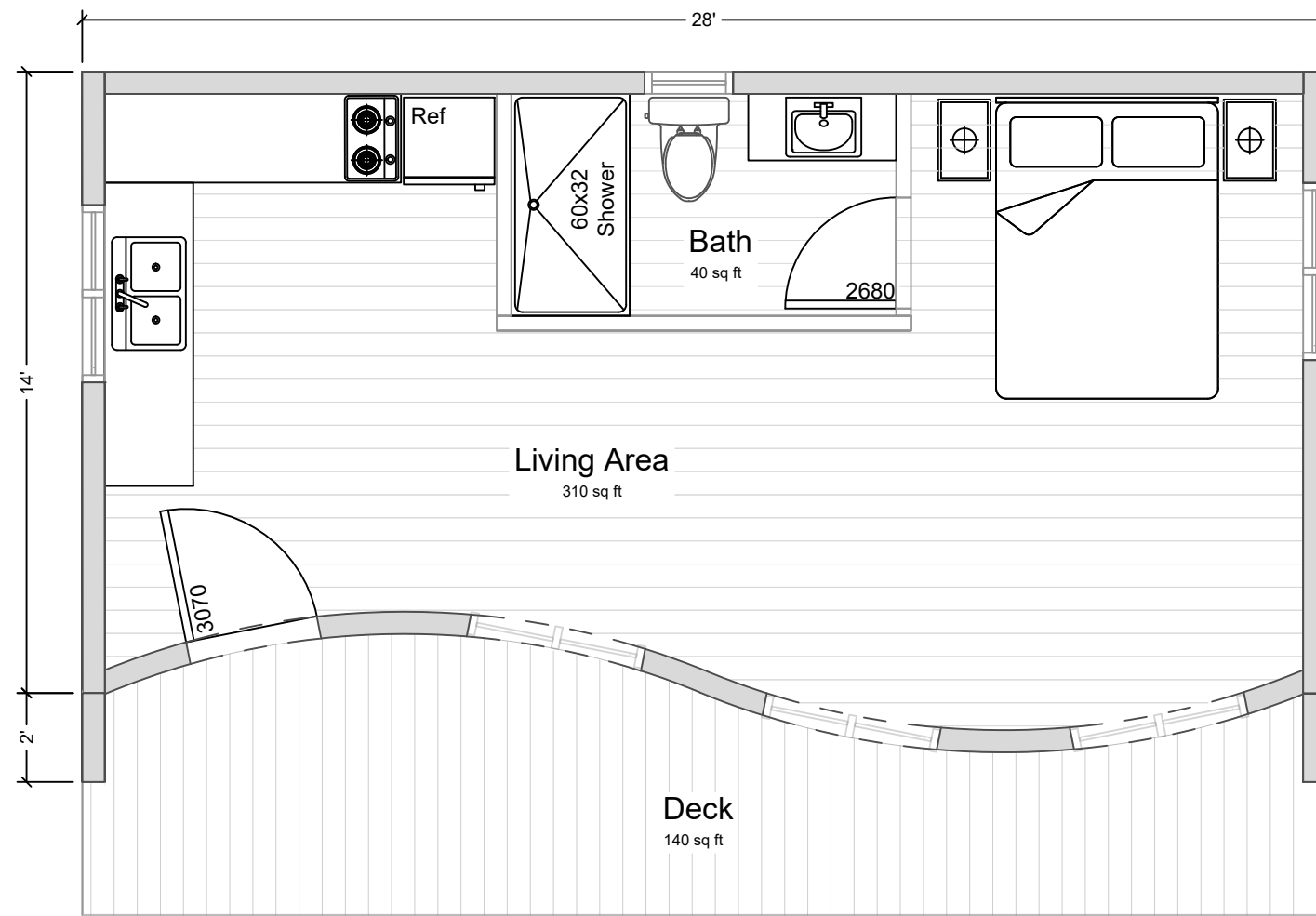
Point Grace 28x14
